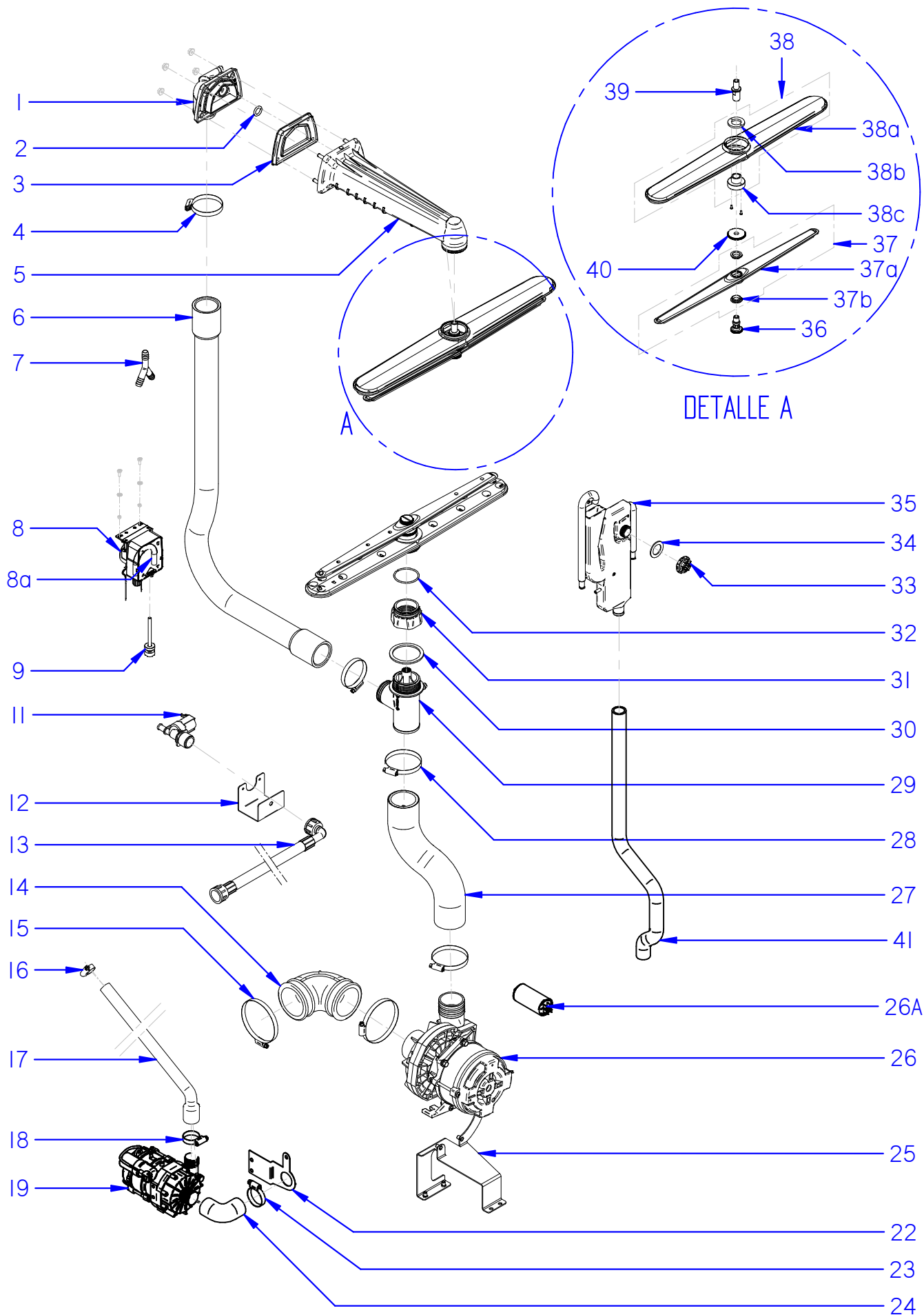
Conjunto hidráulico / Hydraulic assembly – GLB0071/FN / GLB0080N / GLB0082N
