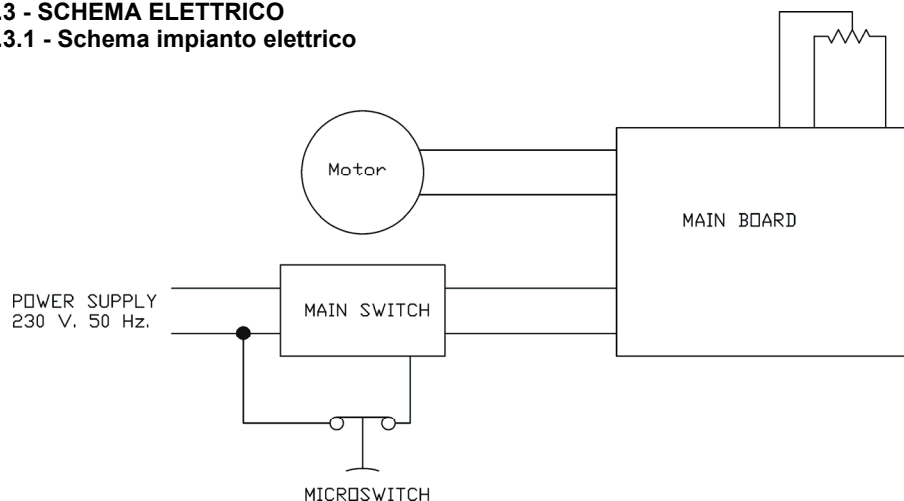
FIG. n°5 - Schema elettrico
